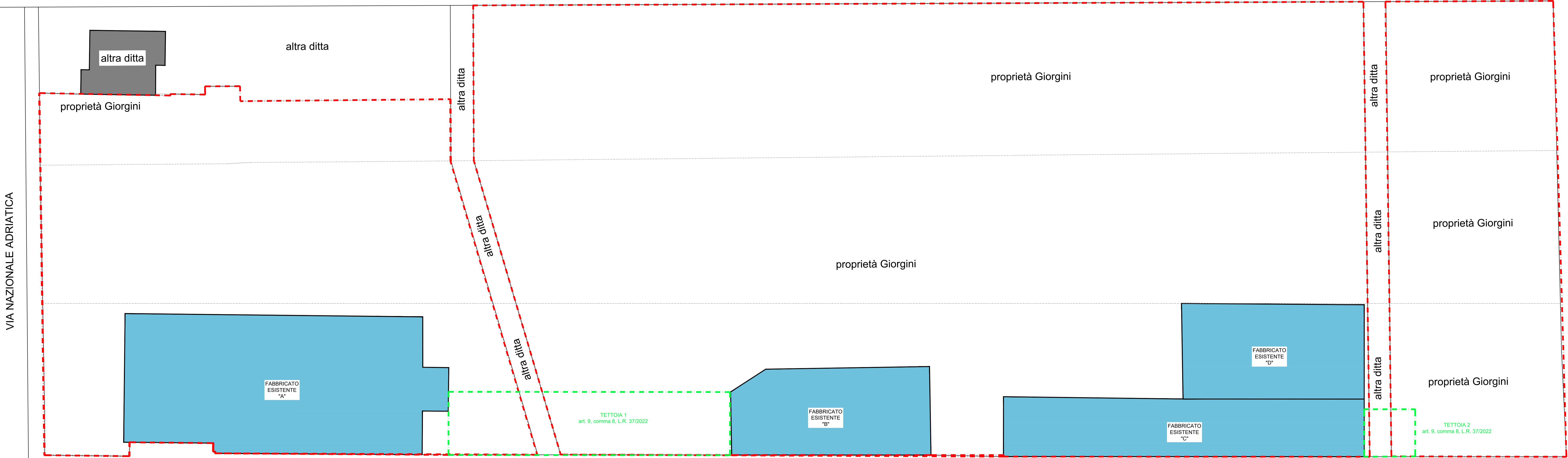
STATO DI FATTO scala 1:200
